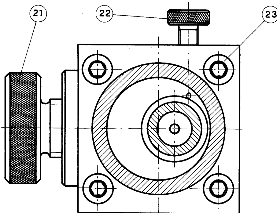
SEZ. A-A
